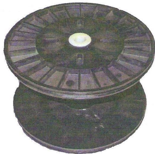
Panter = 3529001P Dornier = 327286D Øe = 213mm -- Øi = 59mm Li = 100mm -- Hole = Ø16mm
