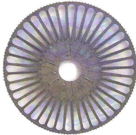
2548096.1 Vamatex - P1001 - VA157 D.361 x D.60 - Z=136
