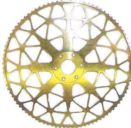
B88372 Picanol - GTX-220 D.379 x D.45 - Z=93
