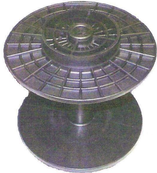
AM8116A Somet Excel - Alpha Øe = 210mm -- Øi = 39mm Li = 150mm -- Hole = Ø20mm
