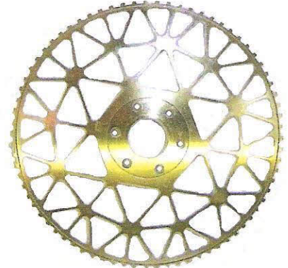
B88251 Picanol - GTM - GTX D.306 x D.45 - Z=75
