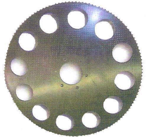
2558276 Vamatex - Leonardo - VA175 D.360 x D.60 - Z=136
