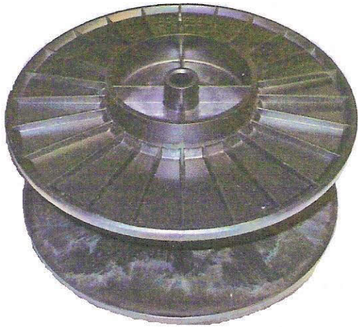
EPS053B Somet Master Øe = 250mm -- Øi = 58mm Li = 83mm -- Hole = Ø15mm
